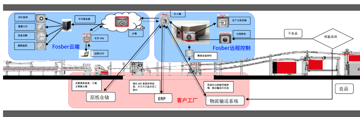
图5：Fosber集团PRO系列智能生产管理信息化系统工作示意图
